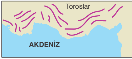
Boyuna Kıyı
