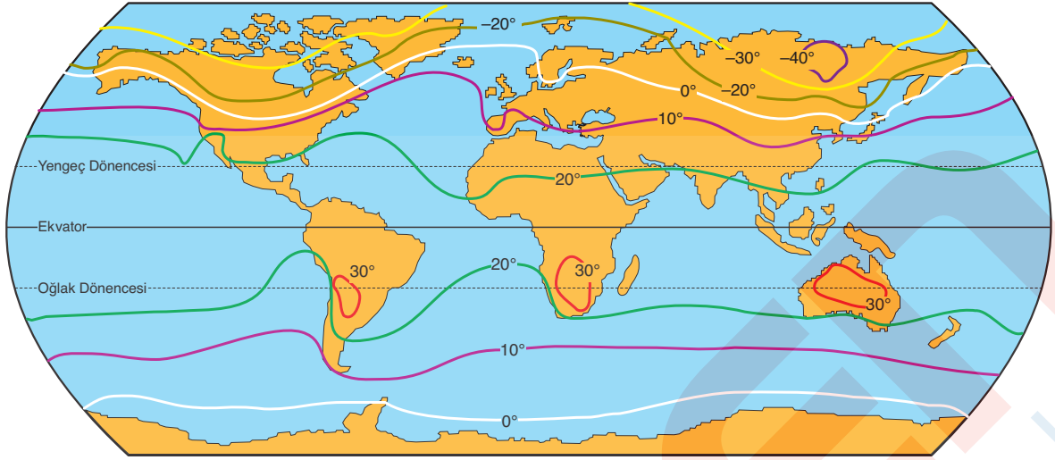
Dünya Ocak Ayı İzoterm Haritası
