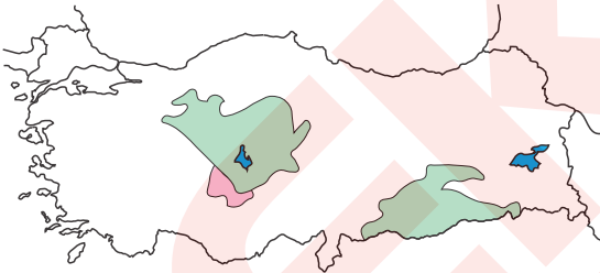
Türkiye'de rüzgar etkilerinin görüldüğü başlıca alanlar.
