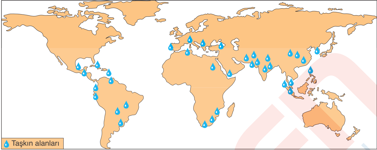
1965 - 1994 tarihleri arasında Dünya'da meydana gelen sel ve taşkınların dağılışı
