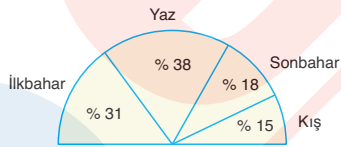
Kars'ta yıllık yağışın mevsimlere göre dağılışı oranı
