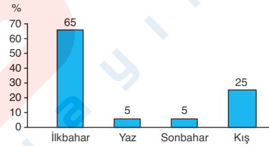
Türkiye’de heyelanın mevsimlere göre dağılışı
