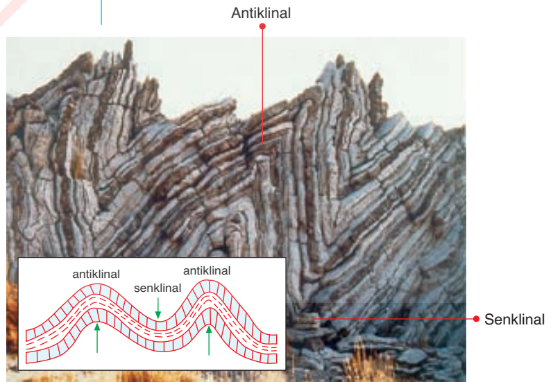
Kıvrımlı yapı
