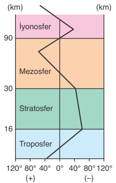
Atmosfer katmanlarındaki sıcaklık ortalamaları
