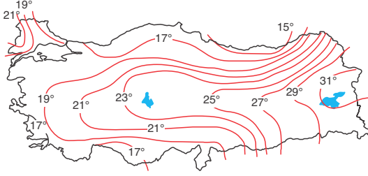
Türkiye'de yıllık sıcaklık farklarının dağılışı
