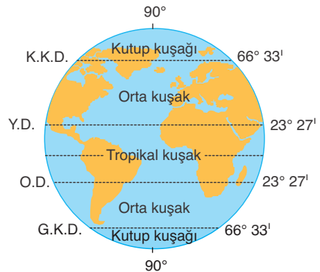
Matematik iklim kuşakları
