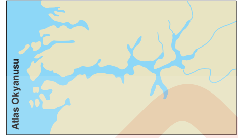
Fiyortlar buzul vadilerinin sular altında kalmasıyla oluşur.
