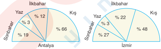
Antalya ve İzmir'de yıllık yağışın mevsimlere göre dağılışı oranı
