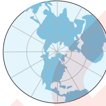
Düzlem projeksiyon
