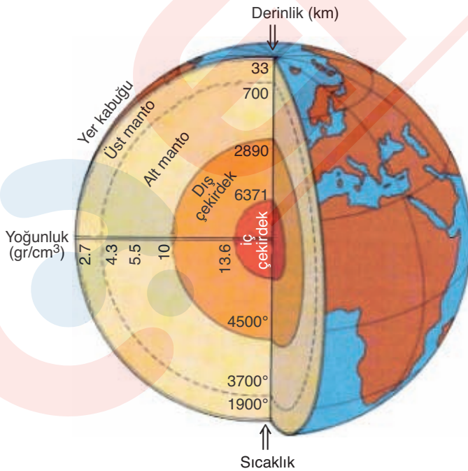
Yer yuvarlağının yapısı
