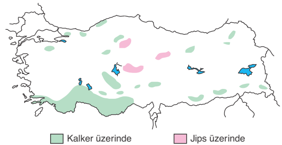
Haritada yurdumuzdaki karstik yöreler gösterilmiştir.
