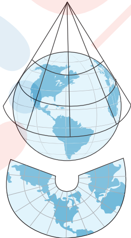
Konik projeksiyon
