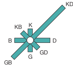
Rüzgar frekans gülü
