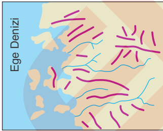
Enine Kıyı
