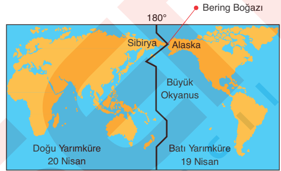
Tarih değiştirme çizgisinin yeri
