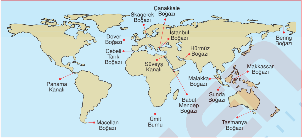
Yeryüzündeki önemli boğazlar
