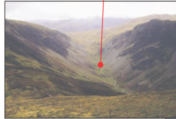
Dik yamaç
