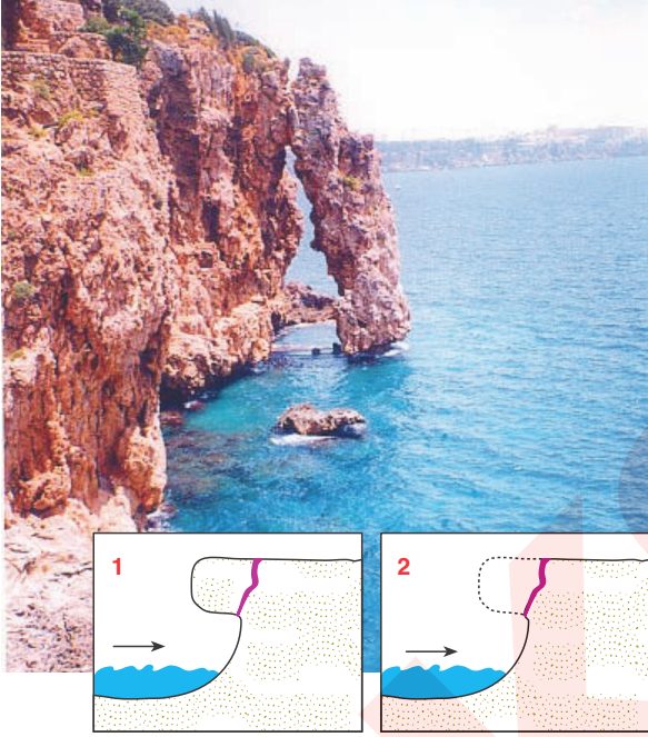
Falez (Yalıyar) Oluşumu
