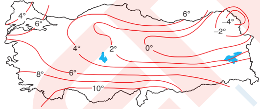
Türkiye'nin Ocak ayı sıcaklık ortalamalarına göre indirgenmiş izoterm haritası
