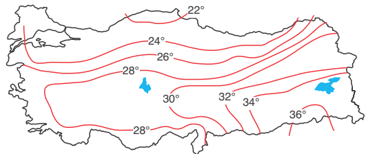
Türkiye'nin Temmuz ayı sıcaklık ortalamalarına göre indirgenmiş izoterm haritası
