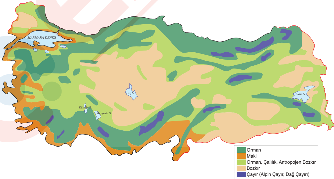
Türkiye'nin bitki örtüsü haritası
