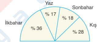
Ankara'da yıllık yağışın mevsimlere dağılışı oranı
