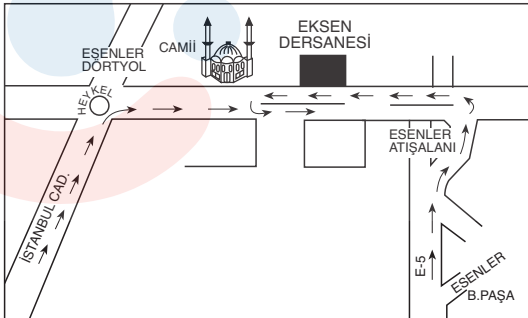
Kroki
