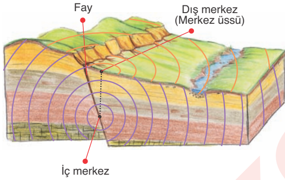
Bir depremin iç ve dış merkezi ile deprem dalgalarının yayılışı
