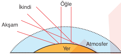
Güneş ışınlarının yeryüzüne düşme açısının günün saatine göre değişmesi
