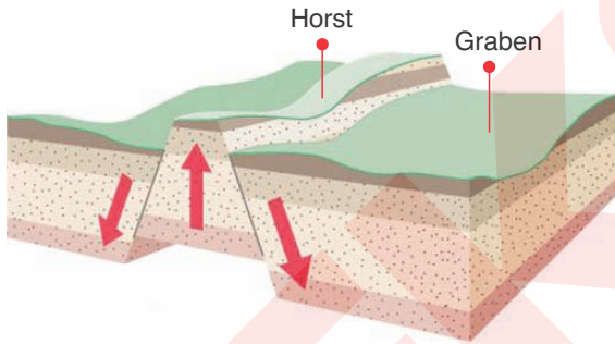
Fay hatları boyunca oluşan horst ve grabenler
