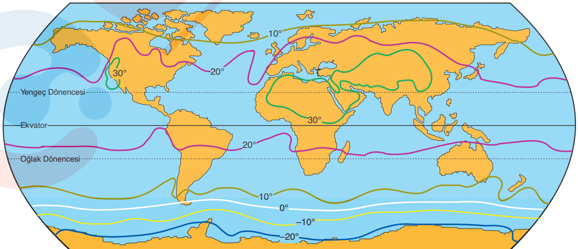
Dünya Temmuz Ayı İzoterm Haritası
