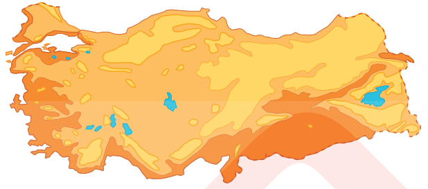
Türkiye'nin temmuz ayı sıcaklık ortalaması haritası
