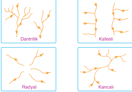
Drenaj Tipleri
