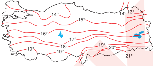
Türkiye'nin yıllık ortalama sıcaklıklarına göre indirgenmiş izoterm haritası
