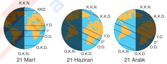
Aydınlanma dairesinin üç farklı tarihteki konumu
