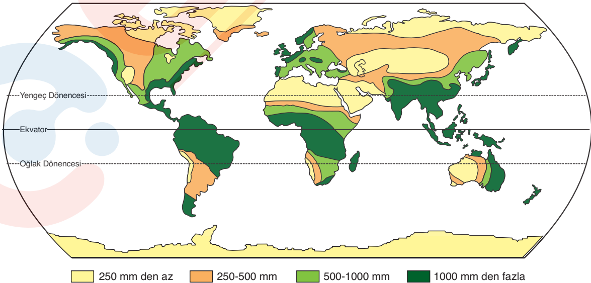
Dünya'nın Yağışlı ve Kurak Bölgeleri
