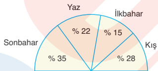
Rize'de yıllık yağışın mevsimlere göre dağılışı oranı
