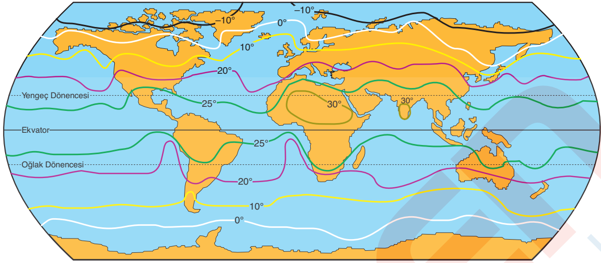
Dünya Yıllık İzoterm Haritası
