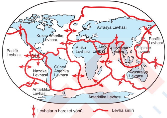
Yerkabuğunu oluşturan başlıca levhalar ve hareket yönleri
