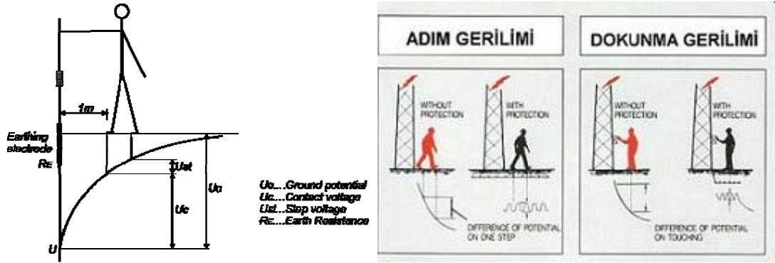
Şekil 10 Adım ve dokunma gerilimi
