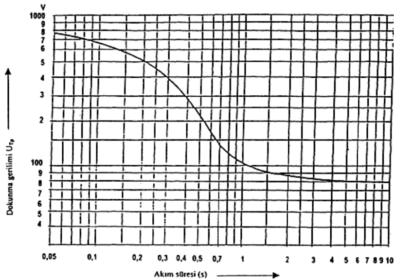
Şekil 10 Adım ve dokunma gerilimi
