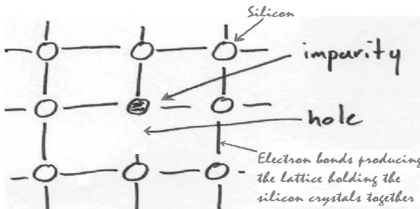
Şekil 4 Yarıiletkenlerde elektron delikleri
